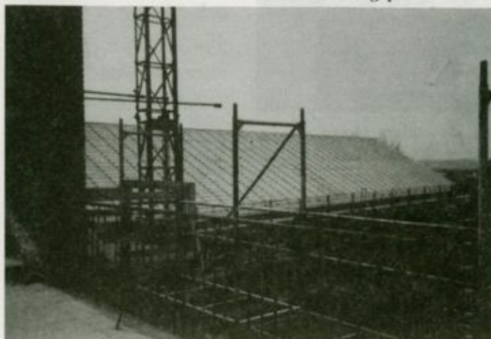
Összeállítás előtt a tetőszerkezet elemei
